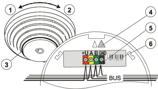
Abb. 6: 1 – Öffnung der Melderabdeckung (entfernen); 2 – Schließung der Melderabdeckung (einsetzen); 3 – optische Anzeige; 4 – Pfeile, zeigen die Stelle, an der der Melder in die Bodenplatte gesteckt werden muss; 5 – Bus-Anschlussklemmen; 6 – Produktionscode
