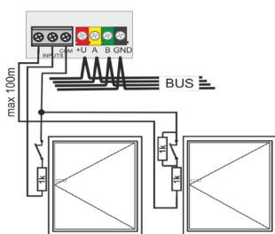
Abbildung 3: Schleifenausgleich
